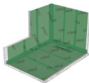
APLICAÇÃO DA TELA IMPERMEABILIZANTE ISOL NAS PAREDES
