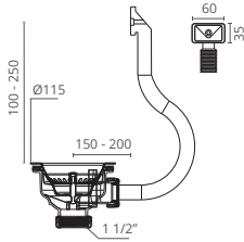
VÁLVULA C/ CESTO INOX E AVISADOR
