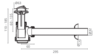
SIFÃO GARRAFA LAVATÓRIO
