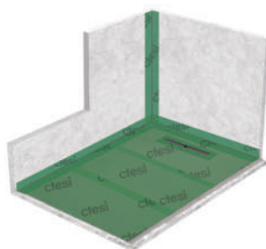
APLICAÇÃO DA TELA IMPERMEABILIZANTE ISOL NO CHÃO
