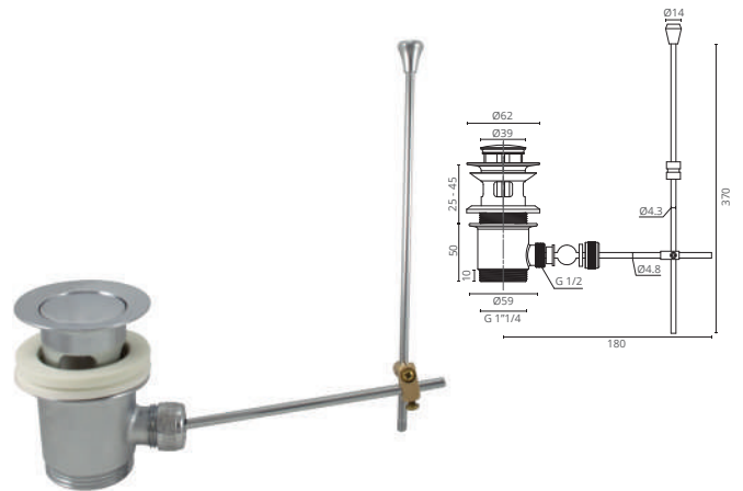
VÁLVULA LAVATÓRIO AUTOMÁTICA C/ VARETA
