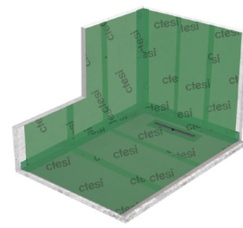
Aplicação da tela impermeabilizante ISOL nas paredes
