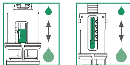
AJUSTE PARA CIMA PARA DESCARREGAR MENOS ÁGUA
